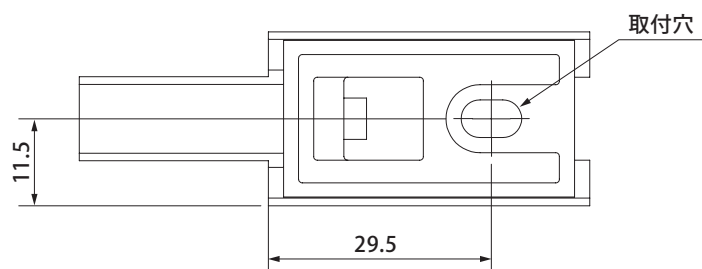
ハイタイプ底面 (尺度1:1)
