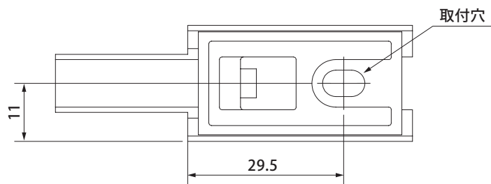
ロータイプ底面 (尺度1:1)
