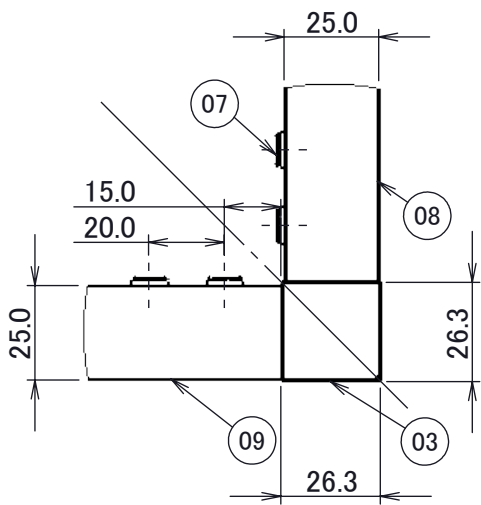
詳細図 B スケール 1 : 2
