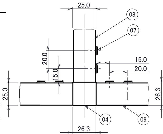
詳細図 C スケール 1 : 2
