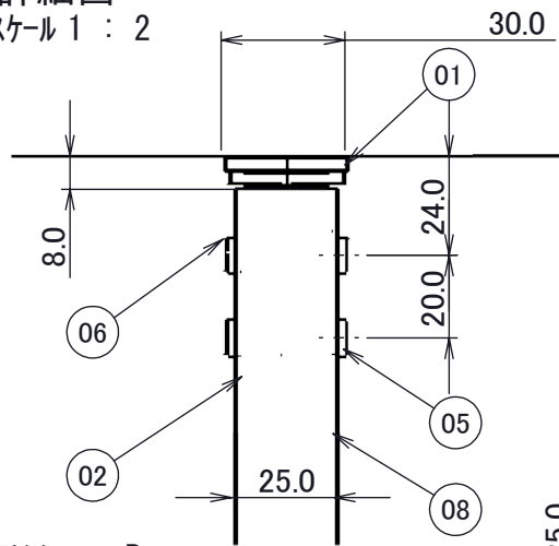
詳細図 B スケール 1 : 2
