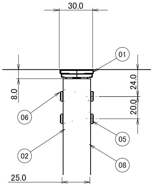
詳細図 A スケール 1 : 2
