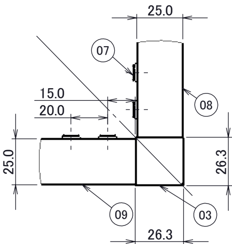
詳細図 D スケール 1 : 2
