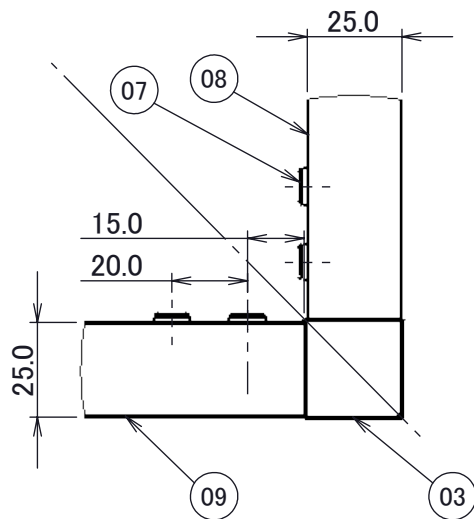
詳細図 C スケール 1 : 2
