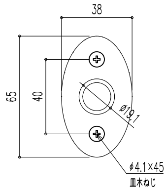
A-A矢視図 (S=1/2)
