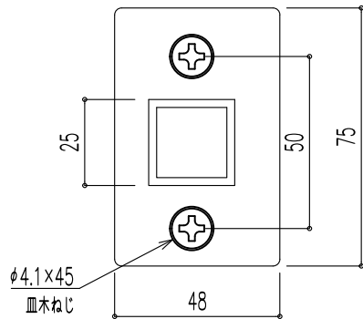
A-A矢视图 (S=1/2)
