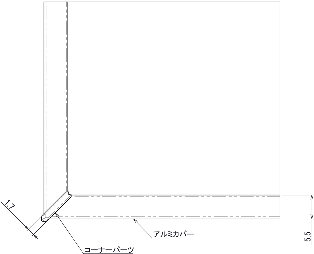
出隅 平面図
