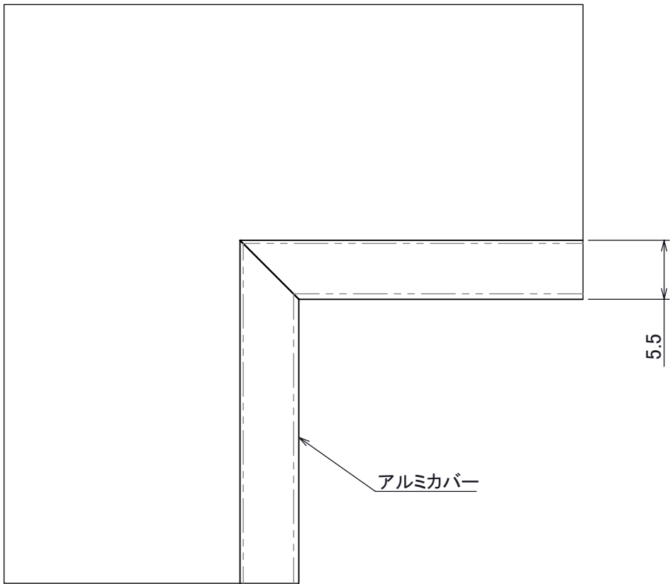
入隅 平面図
