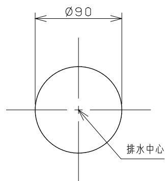
カウンター切込寸法
