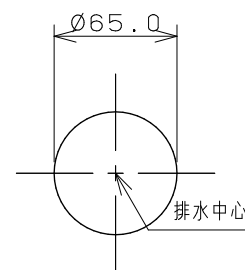
カウンター切込寸法
