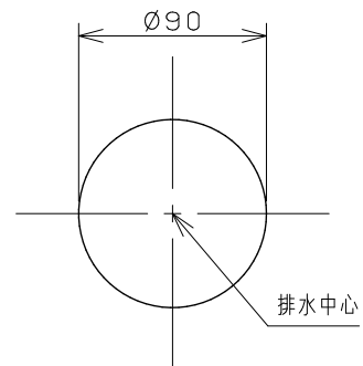
カウンター切込寸法
