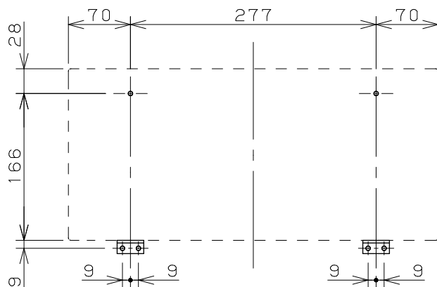
ねじ・固定金具取付位置
